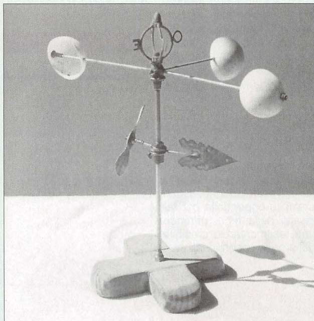
L'anemometro costruito con palline da ping-pong.
