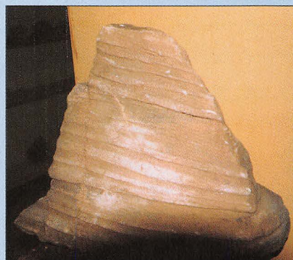
Sez. mineralogia: pietra calcarea corrosa e arricchita da granuli di sabbia calcarea.
