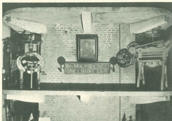
Le due prime macchine che Don Bosco usò quando aprì la prima Scuola grafica salesiana — un torchio a leva e una tagliacarta — sono esposte nel nuovo " Museo delle Arti Grafiche " al Valentino di Torino
