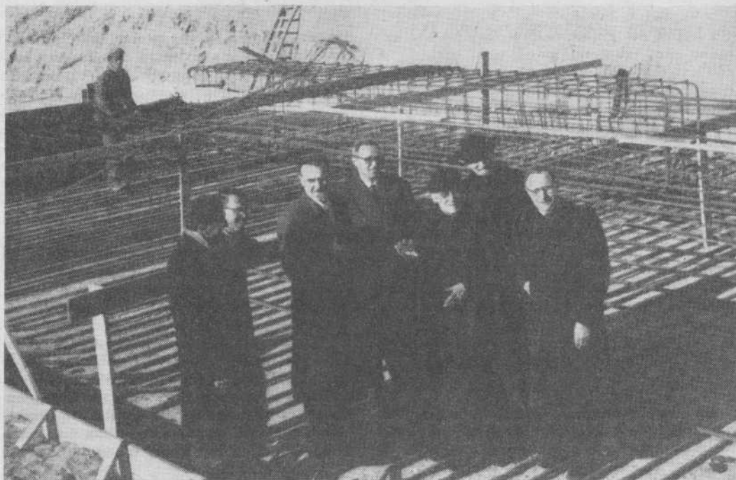
Colle Don Bosco (Asti) - L'Economo Generale, Rev.mo Don Fedele Giraudi, prende visione dei lavori del Tempio a San Giovanni Bosco, all'inizio della posa del ferro di armatura del primo zatterone di fondazione ai campanili
