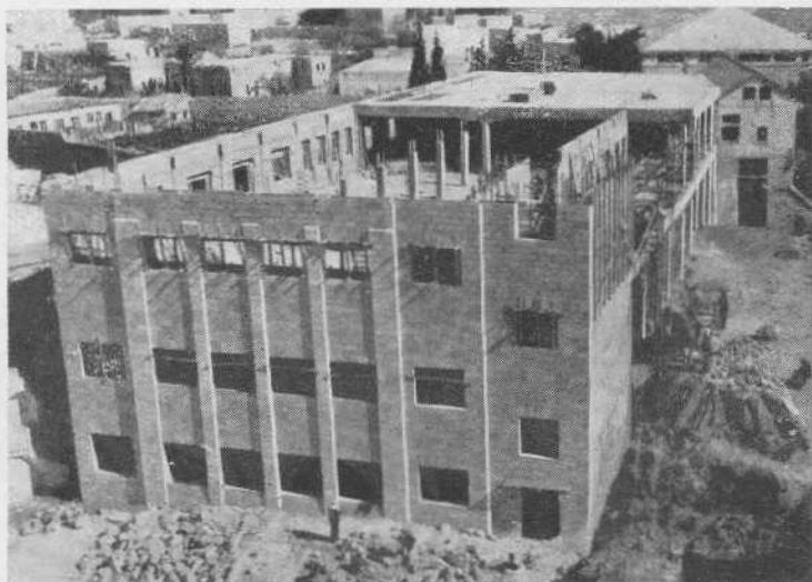
BETLEMME - Il nuovo edificio delle Scuole professionali salesiane in costruzione.
