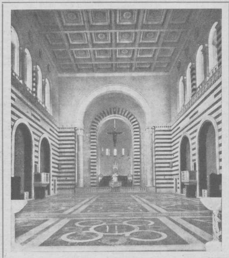
GENOVA-SAMPIERDARENA - Nuovo tempio a S. Giovanni Bosco. « Non ho voluto fare — dichiara l'ing. Pietro Stura, progettista — una chiesa romanica, né gotica, né 900. Ho voluto costruire nel 1955 un edificio che avesse i requisiti di una chiesa ».
