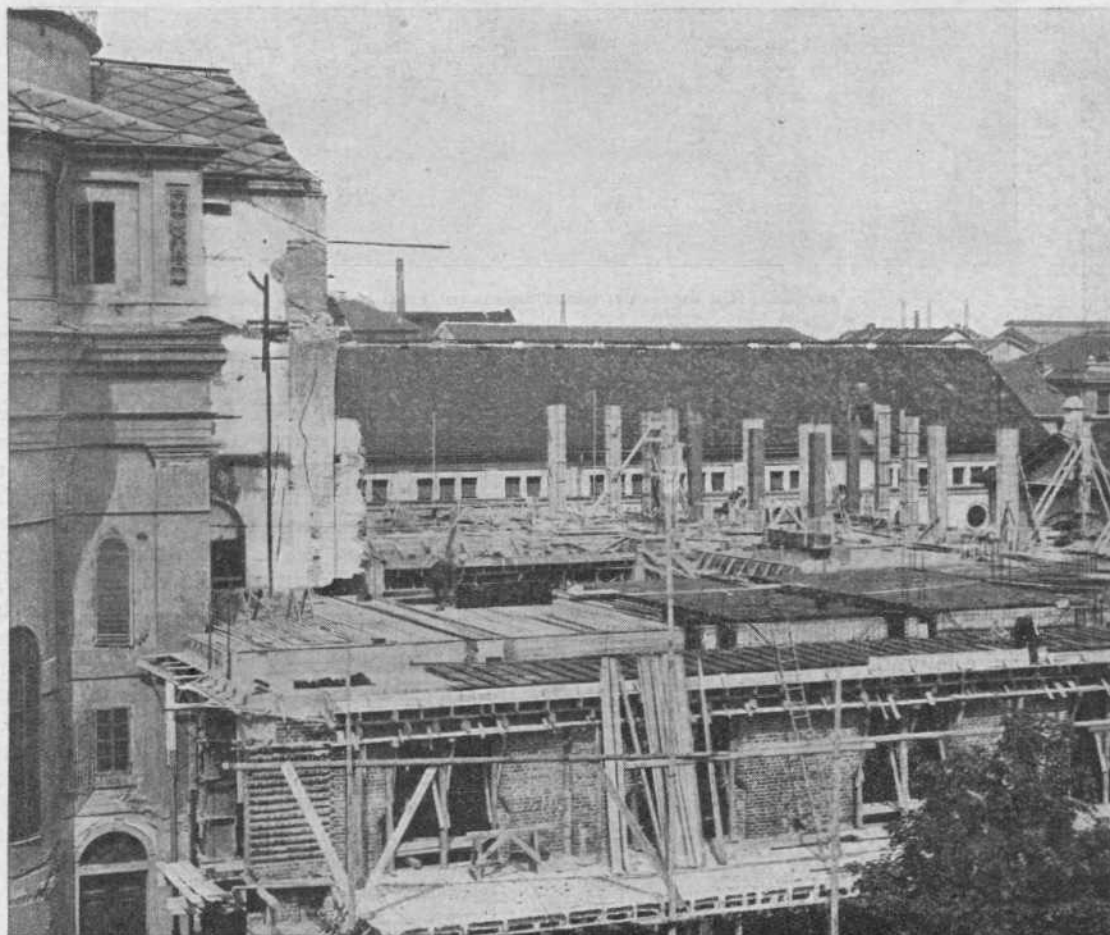
Torino. - L'ampliamento del Santuario di Maria Ausiliatrice. - Lo stato dei lavori in fine di agosto.
