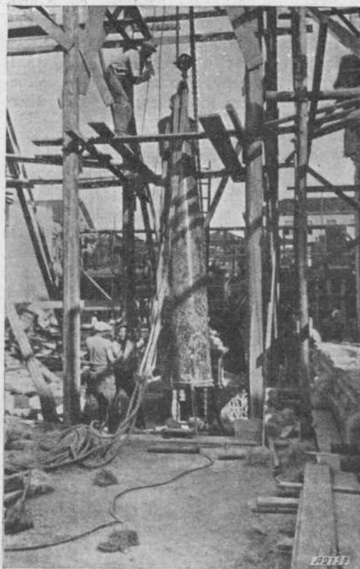
Il collocamento di una delle quattro grandi colonne del presbiterio.
