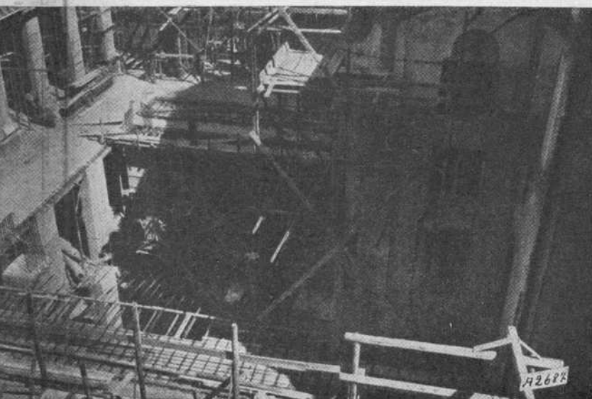
e della pensilina. - Una travata di collegamento delle piastre di fondazione dei pilastri della fondazione. - Veduta dell'interno della zona dei lavori.
