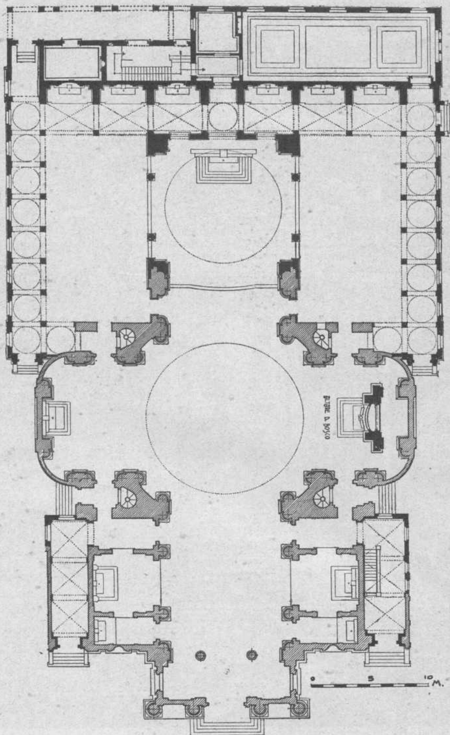
Pianta del Santuario dell'Ausiliatrice.
