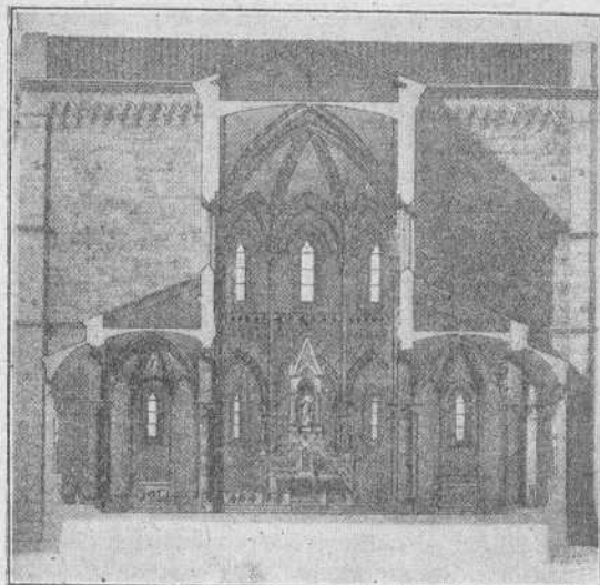
Sezione trasversale.
