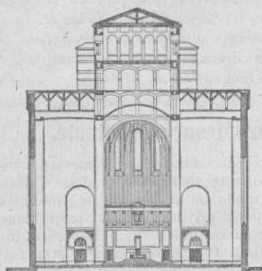
4) Sezione trasversale.
