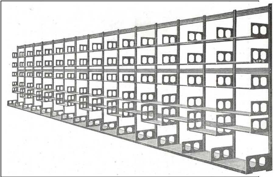
Fig. 4. – Serie di scaffali unilaterali.
