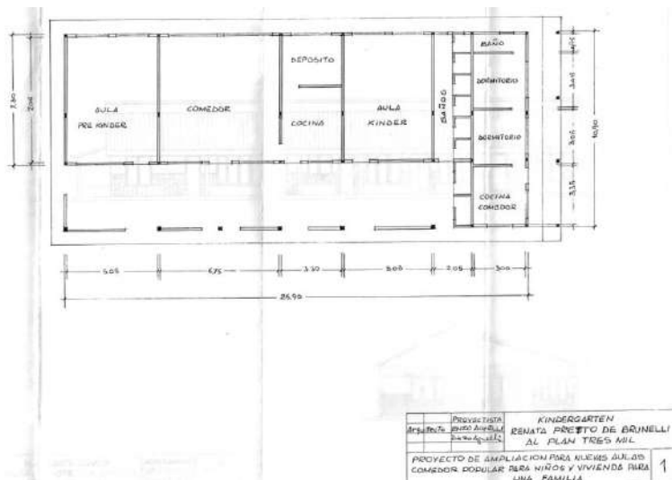
Pianta del progetto di ampliamento del kinder (arch. Enzo Agnelli).
