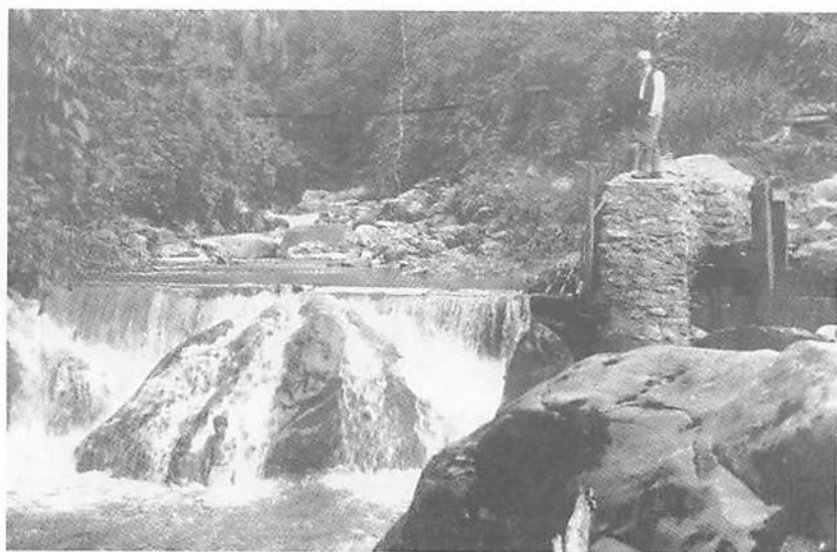
Figura 33. Méndez, Jacinto Pankeri junto a la obra de la presa que debía servir para la central eléctrica (af-cgs).
